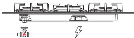
Ansicht Geräterückseite
