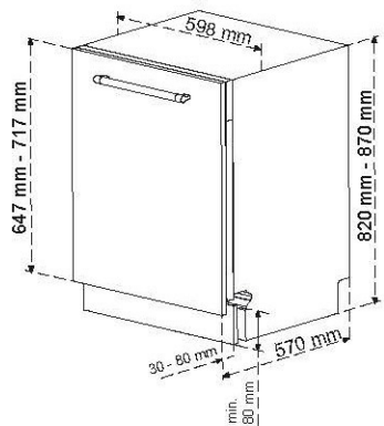
Maßzeichnung GAVI 7582 XL
